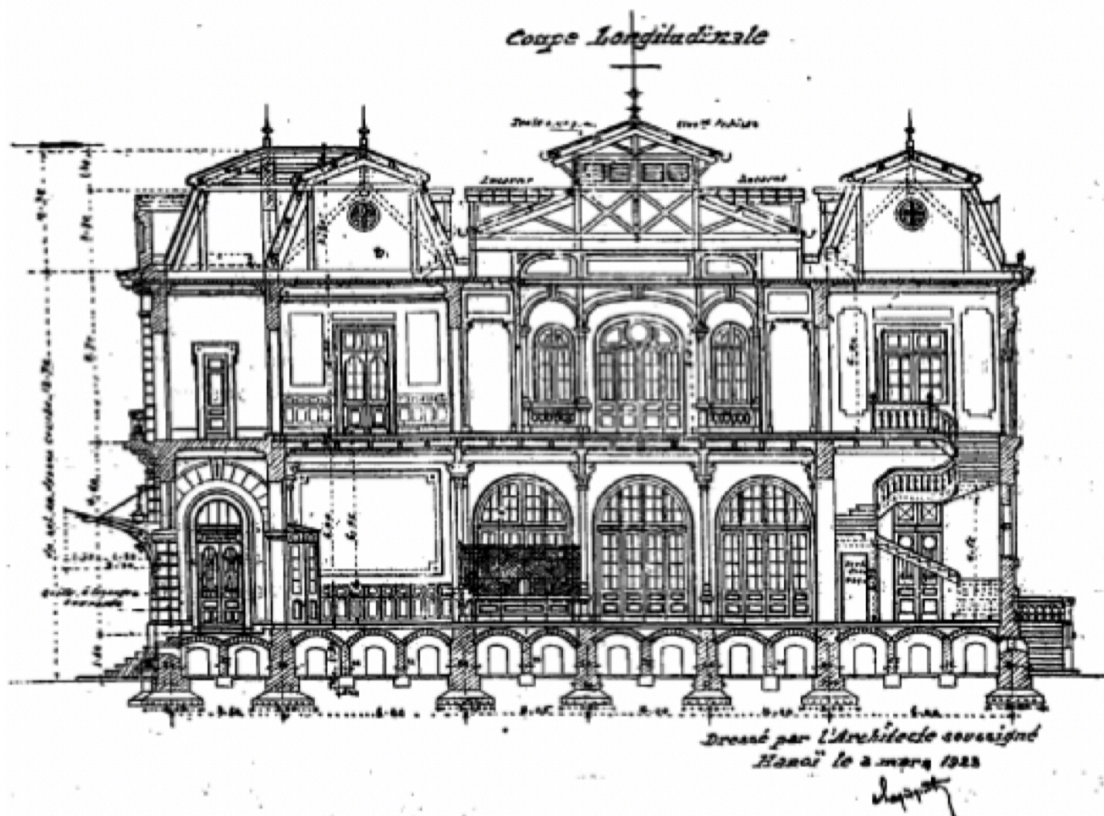
Coupe longitudinale
